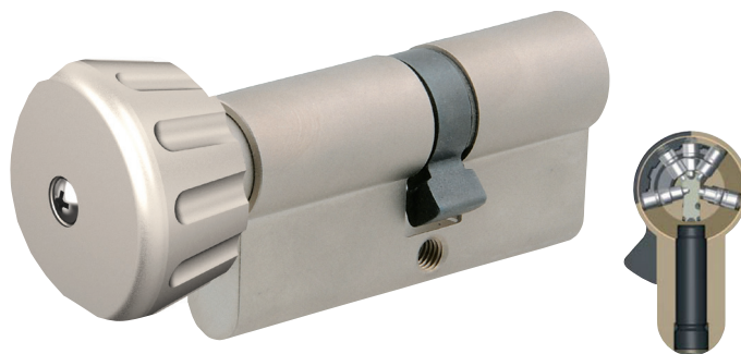
průřez vložky
