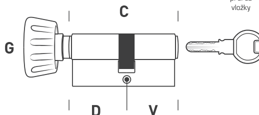
průřez vložky
