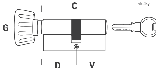
průřez vložky
