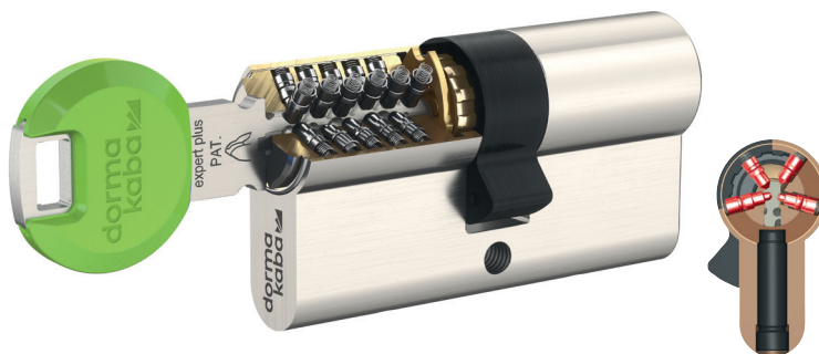
průřez vložky
