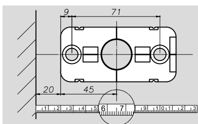
BOHRBILD BODENBEFESTIGUNG
